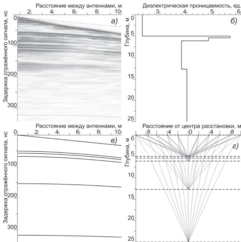
Рис. 3. Результат наклонных зондирований по методу ОГТ, выполненных в пункте R1: a — радарограмма; б — скоростная модель; в — теоретический годограф; г — ход лучей в рамках модели наклонно-слоистой среды. Положение пункта наклонных зондирований показано на рис. 2.
