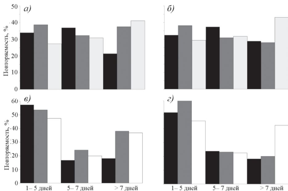
Рис. 2. Частота установления форм циркуляции за период с 1891 по 2015 (а, б) и с 1980 по 2015 гг. (в, г) за холодный (а, в) и теплый (б, г) периоды по градациям: короткие (1–5 дней), средние (5–7 дней) и длинные (более 7 дней) (черный цвет — форма С, серый цвет — форма W, белый цвет — форма E).
