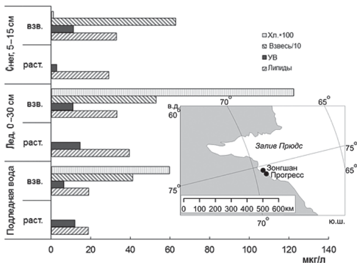
Рис. 1. Распределение органических соединений и взвеси в снежно-ледяном покрове оз. Степед в марте 2012 г.: взв. — соединения во взвешенной, раст. — в растворенной формах.
