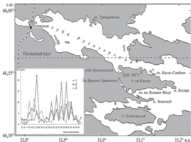
Рис. 3. Схема расположения исследованных отделяющихся озер в губе Ругозерской. На вставке состав алканов донных осадков озер: 1 — Кисло-Сладкое, 2 — на Зеленом Мысу, 3 — Трёхцветное.
